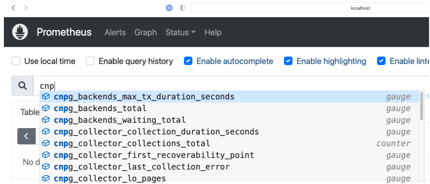
Fig. 8: local prometheus
