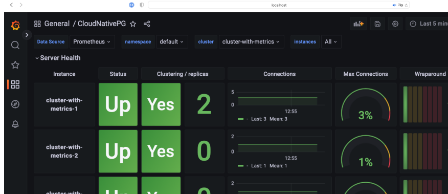
Fig. 9: local grafana
