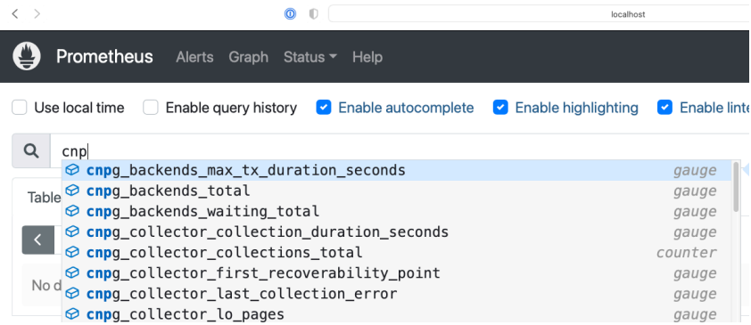
図 9: local prometheus
