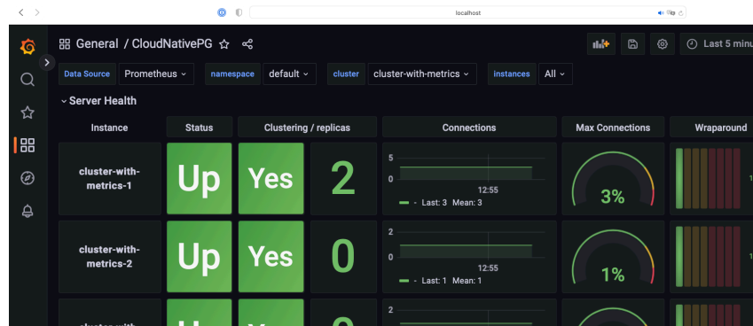
図 10: local grafana
