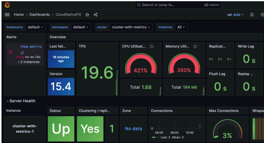
Fig. 2: local grafana
