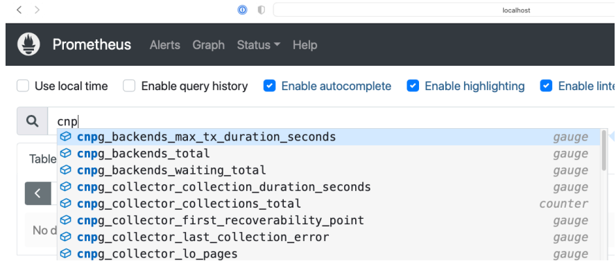
Fig. 1: local prometheus
