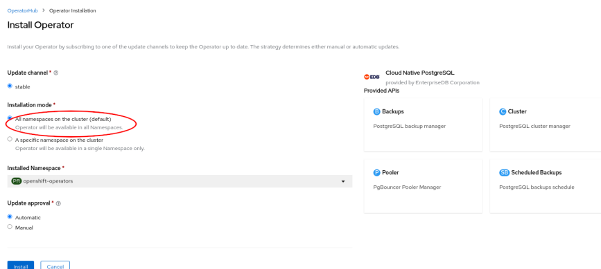
Fig. 4: Install all namespaces
