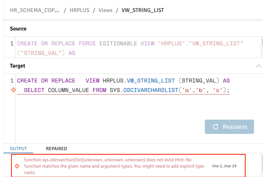
図 5: Syntax error message
