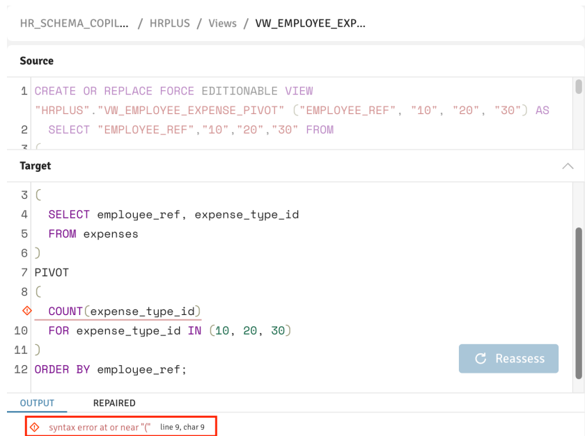
図 6: Imprecise syntax error message
