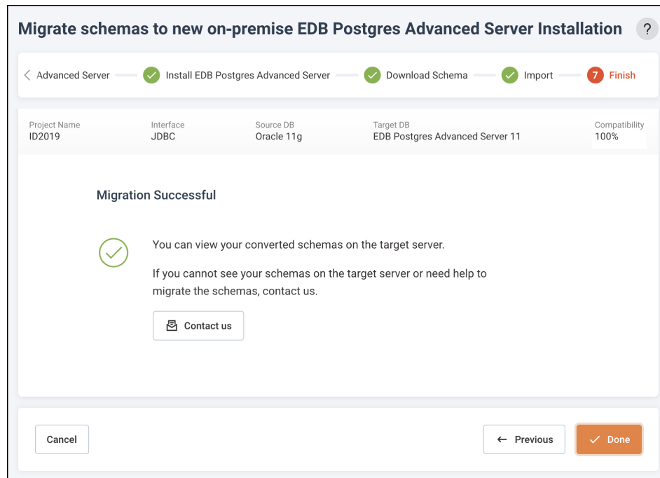
図 38 スキーマ移行の成功
