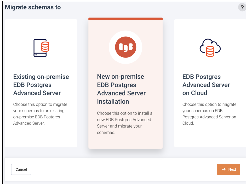
図 31 スキーマのホームページの移行
