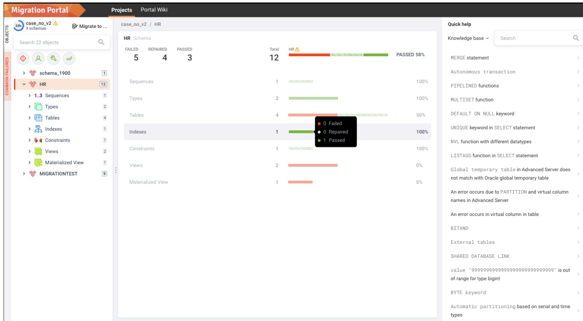
図7 DDL オブジェクトの検証。
