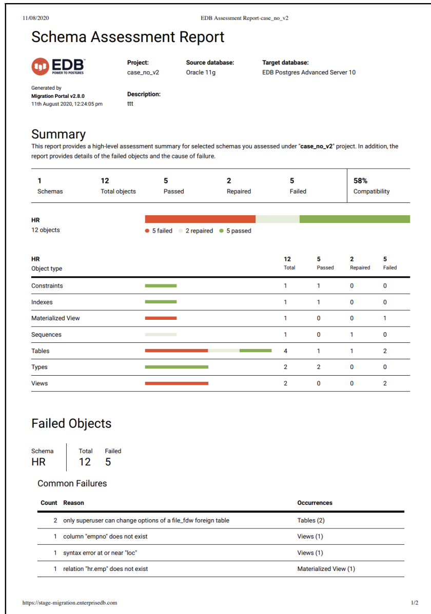
図 13 保存された pdf レポート。
