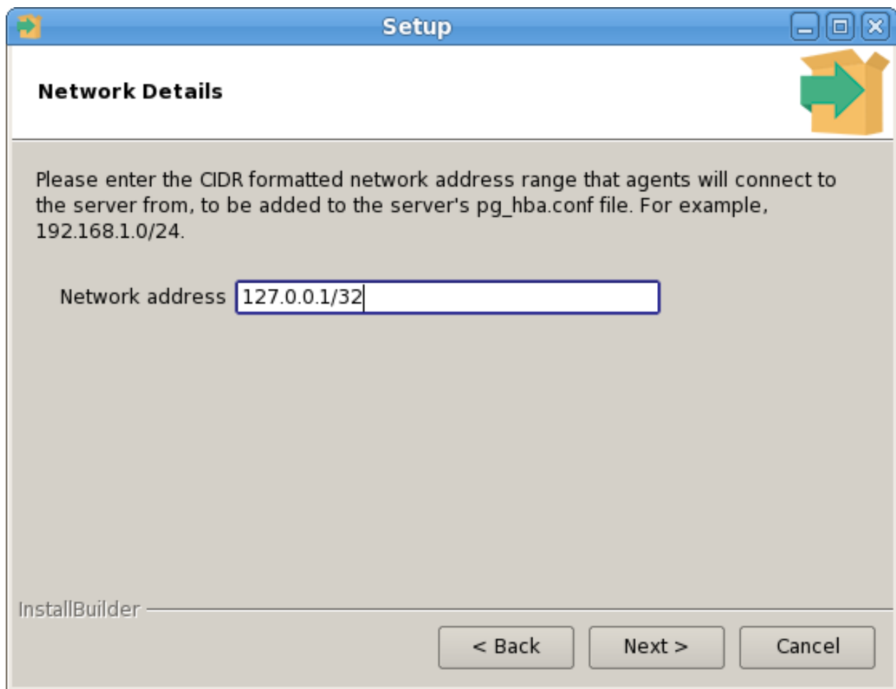
図 37 エージェントが接続するネットワークアドレスを指定します
