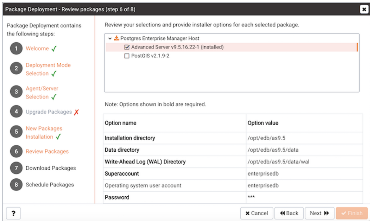
Fig. 5: Specify installation options
