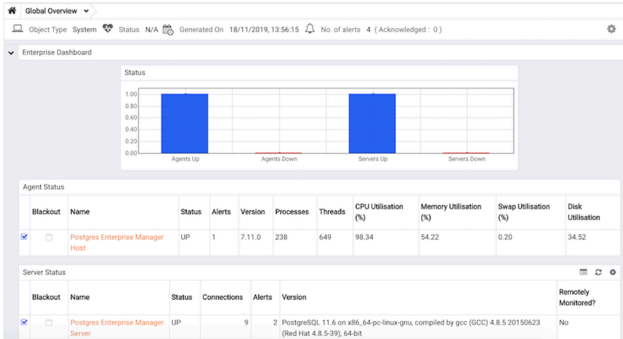
図 3 クライアントに表示されるグローバル概要ダッシュボード
