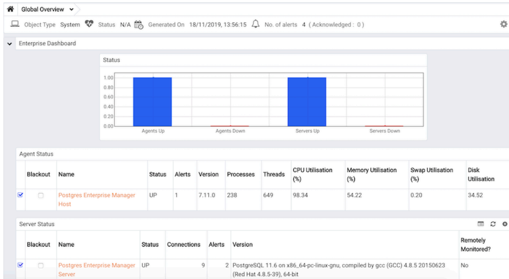
図 11 登録済みサーバー
