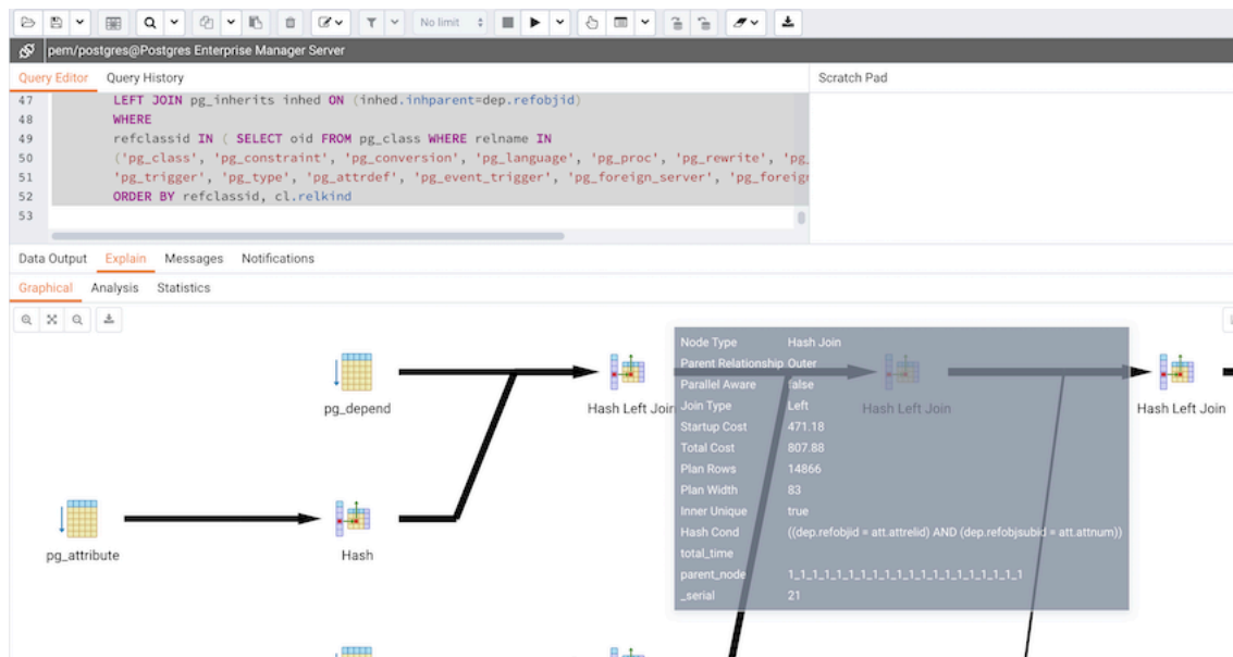
図 10 グラフィカルな説明
