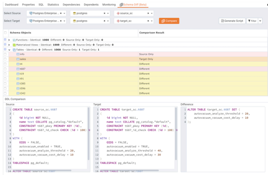
図 1 スキーマ差分ダイアログ
