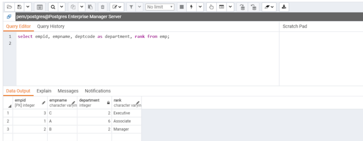
図 8 クエリツールの編集可能な列
