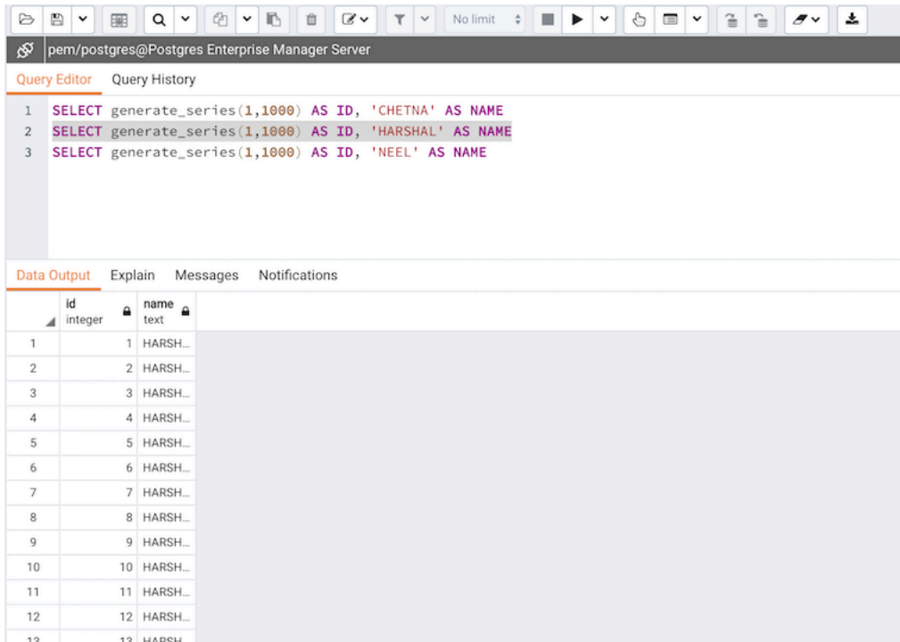
図 5 コマンドの実行
