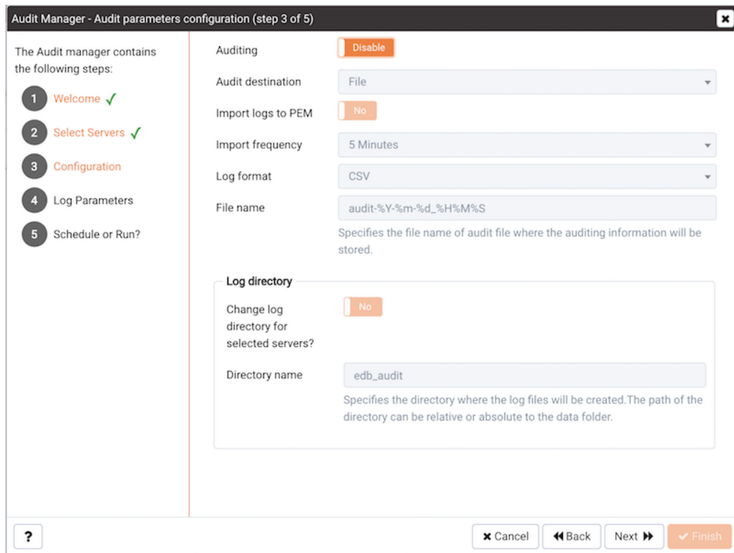
図 5 監査パラメータ設定ダイアログ
