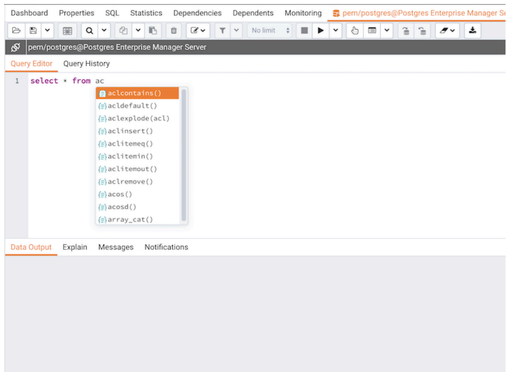
図 4 オートコンプリートを使用する
