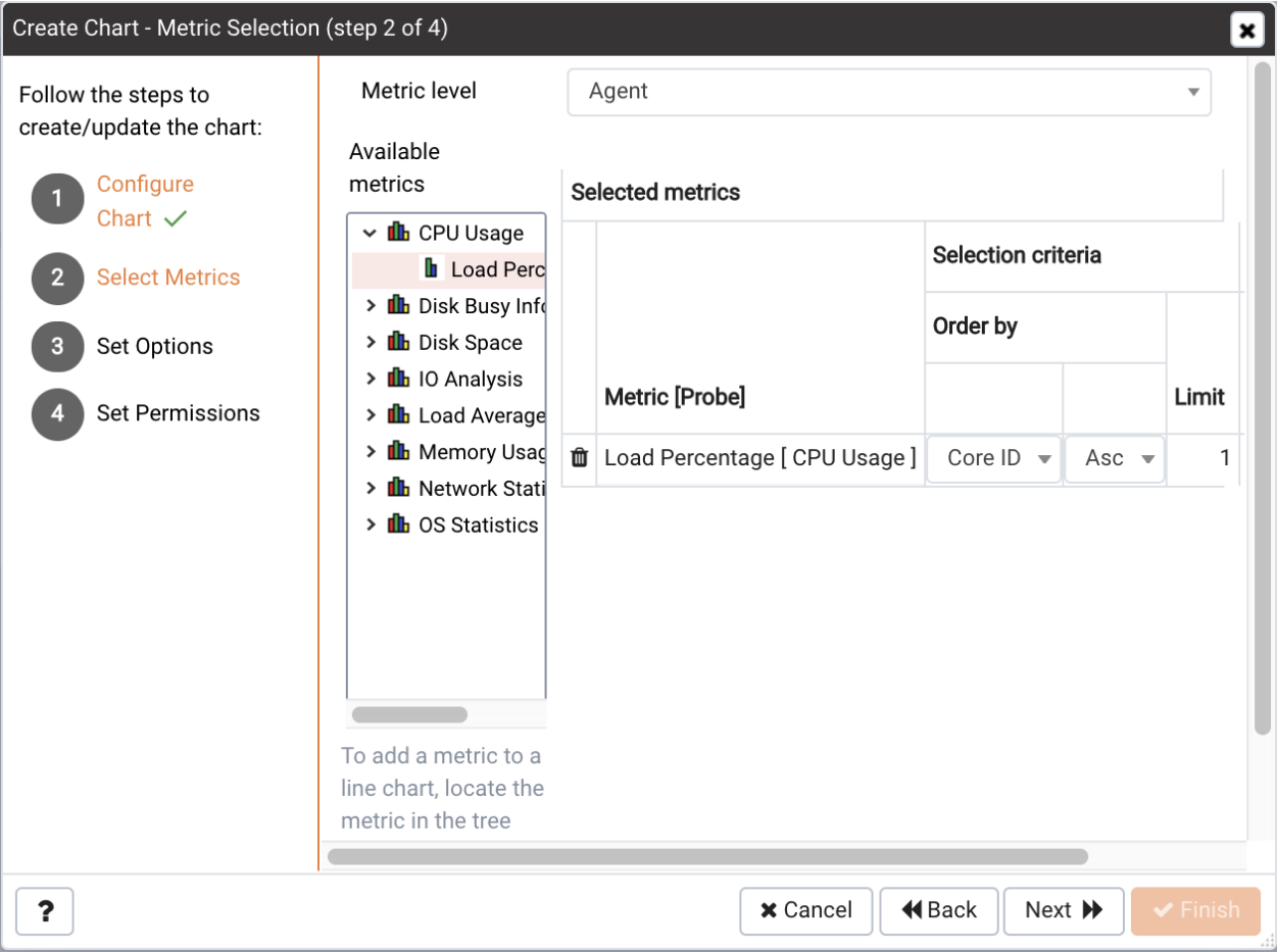
図 12 表示されるメトリックの指定
