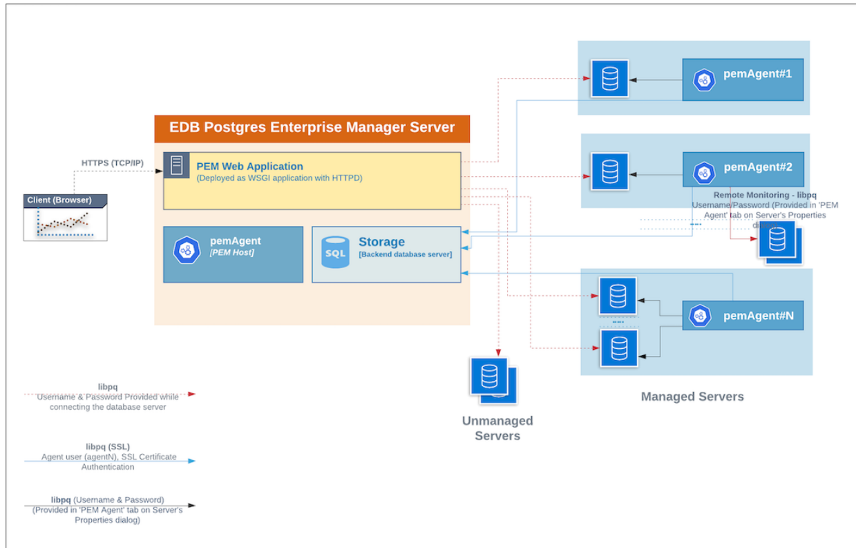
図 1 PostgresEnterpriseManager の一般的なアーキテクチャ
