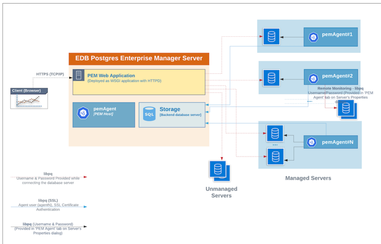
図 1 典型的な PEM インストール。
