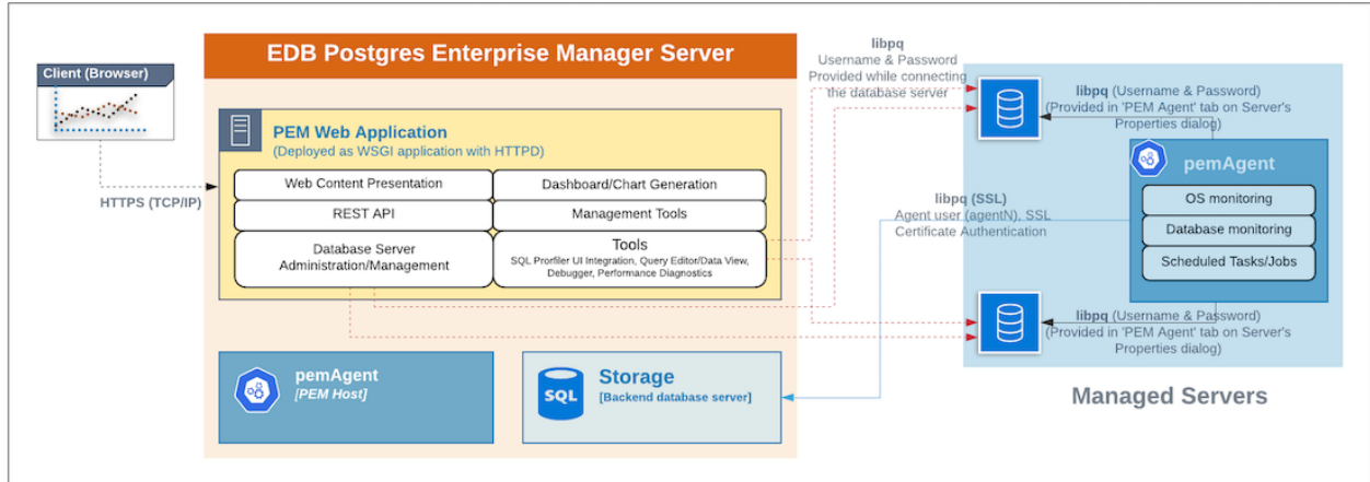
図 3 PEM Agent
