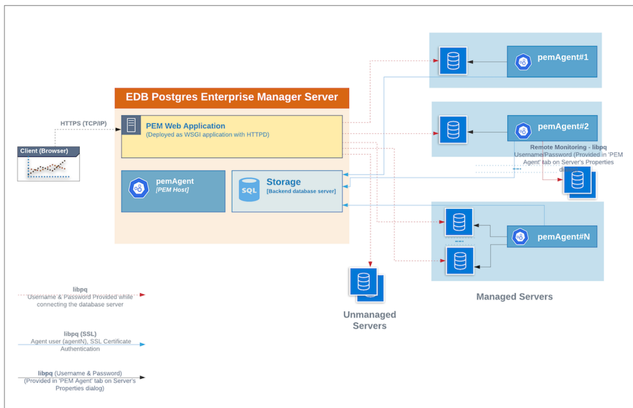
図 1 PEM Architecture
