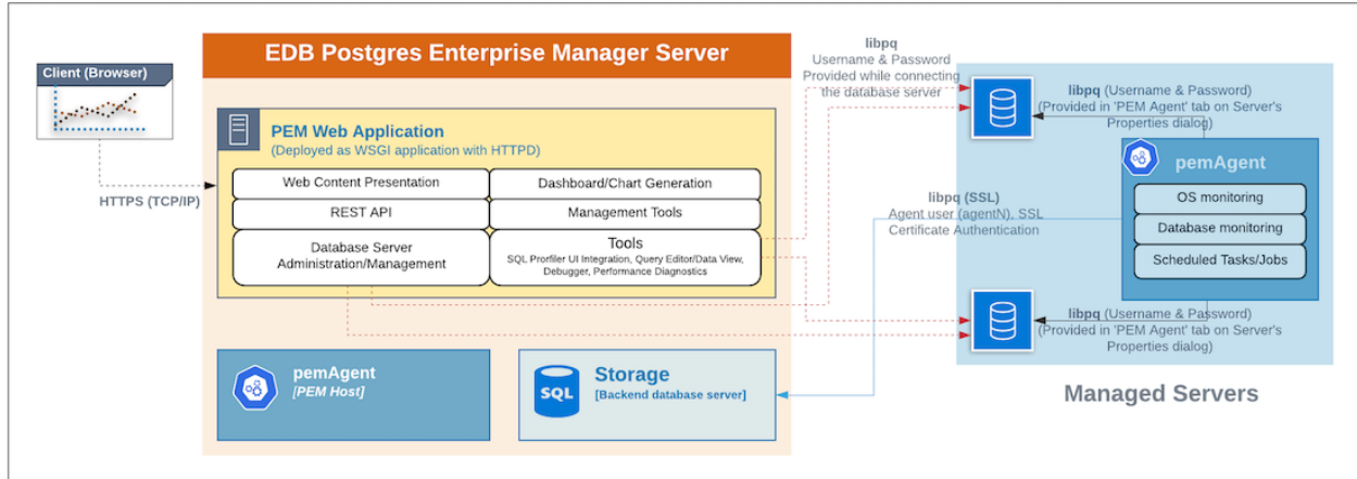
Fig. 3: PEM Agent
