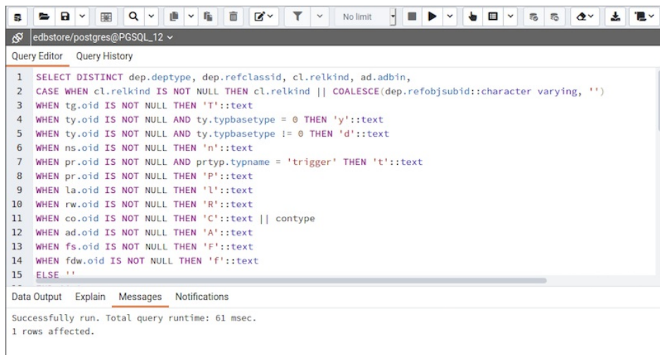
Query Tool - Messages tab
