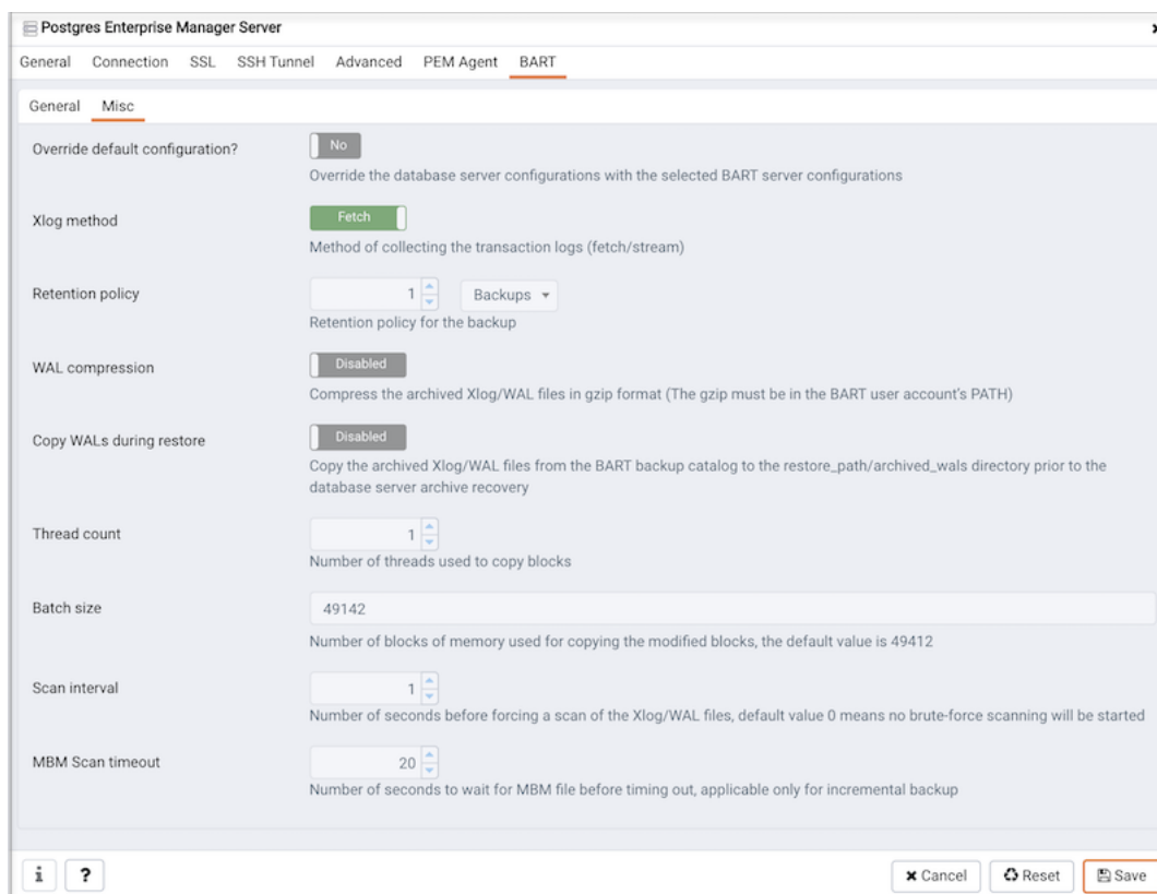
図 10 The Create - Server dialog (BART - Misc tab)
