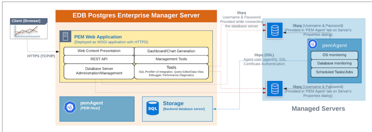
Fig. 3: PEM Agent
