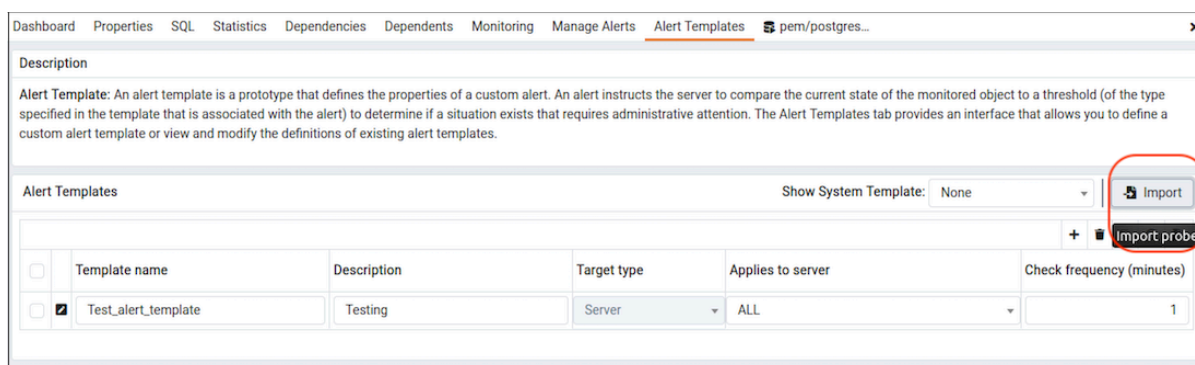
図 46: Alert Templates Import
