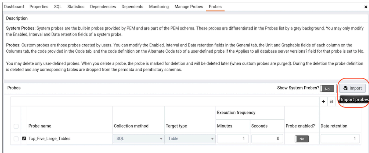
図 28: Custom Probes Import
