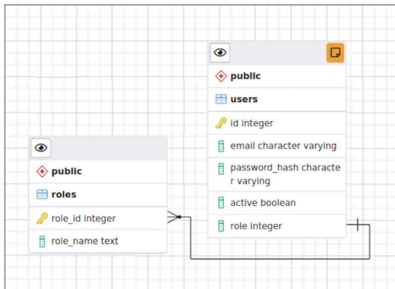
図 7: ERD Tool - Table Link
