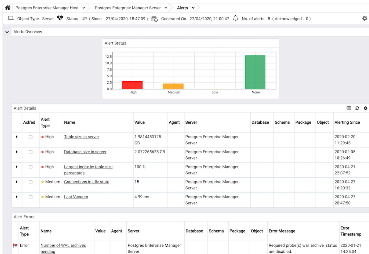
図 37: The Alerts Dashboard
