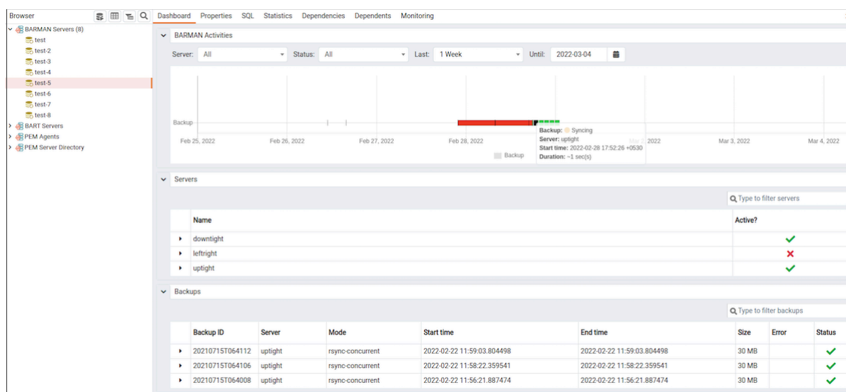
図 1: BARMAN dashboard
