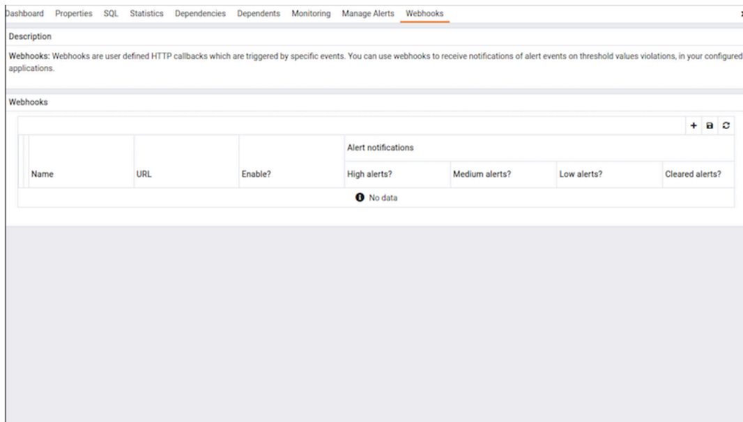
図 70: Webhooks tab
