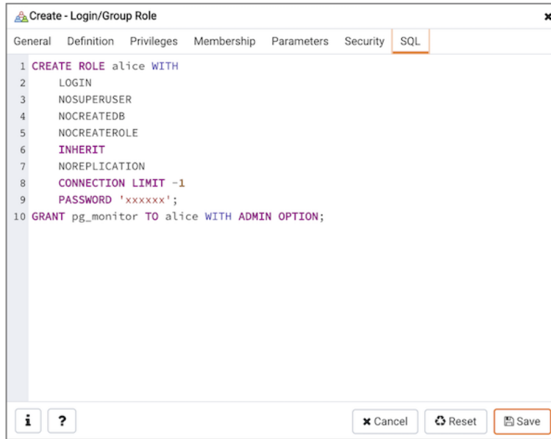
Fig. 8: Create Login Role - SQL tab
